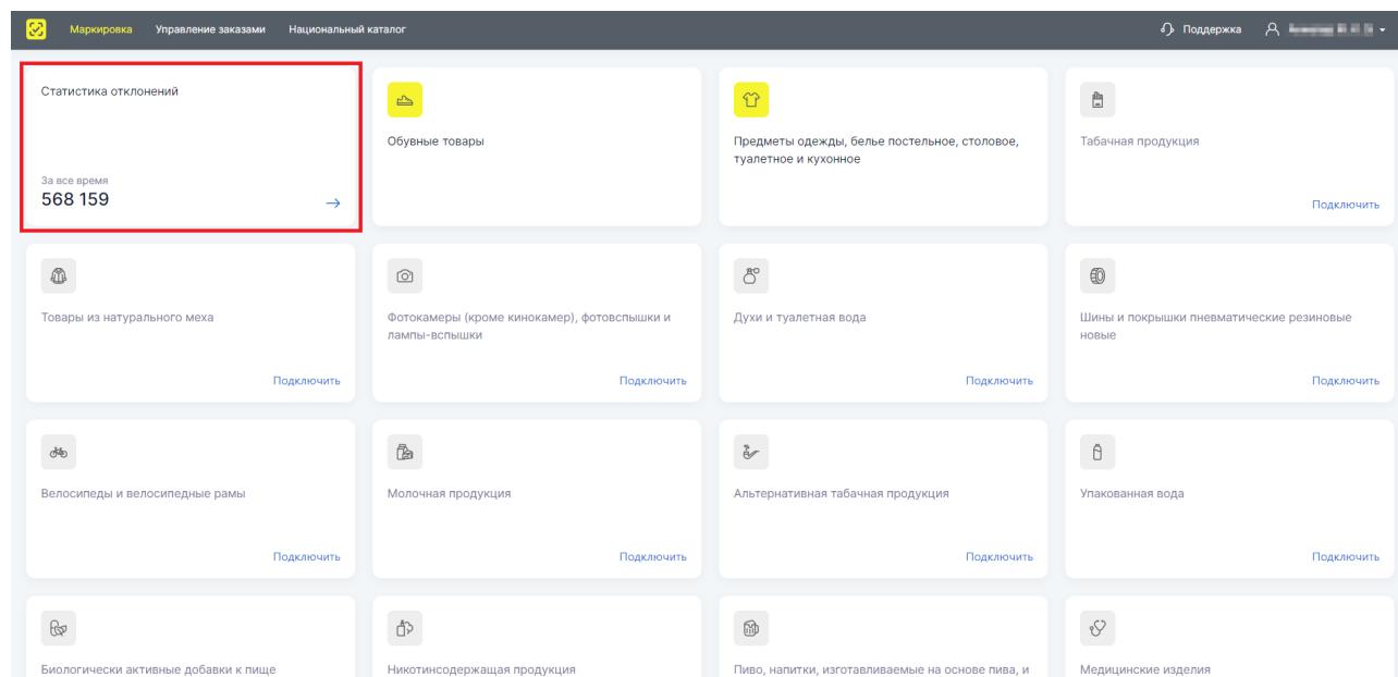
Рисунок 1. Статистика отклонений
